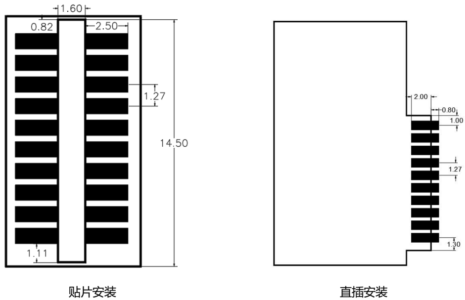
图 5 推荐封装图
