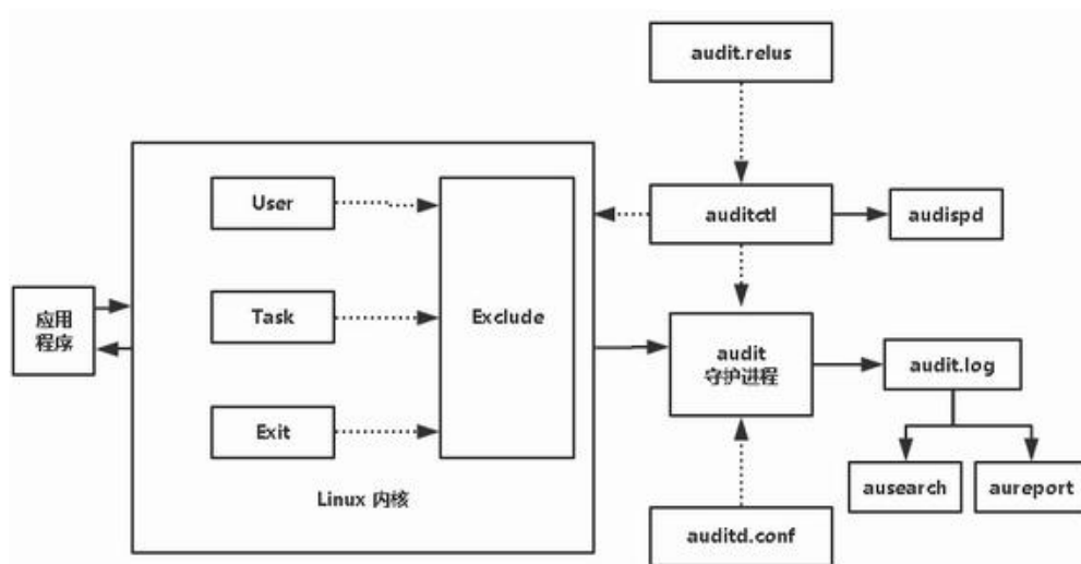
图 8-10 架构示意图
