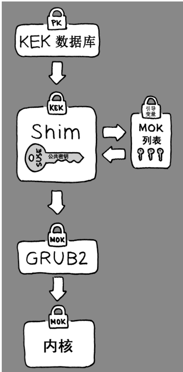
图 11.2 : UEFI: 安全引导流程
