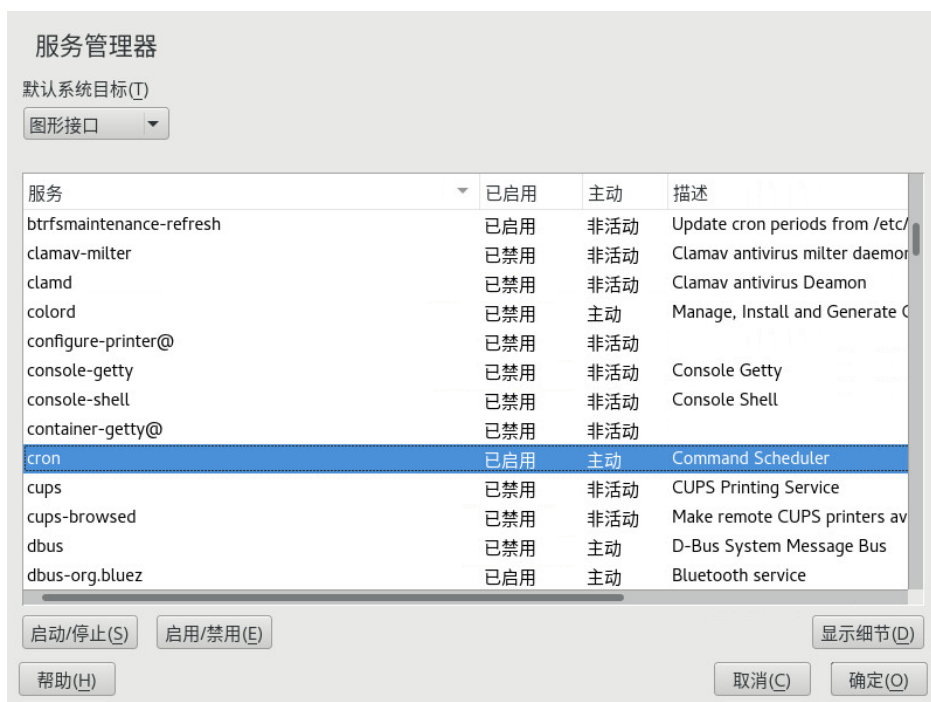
图 13.1：服务管理器
