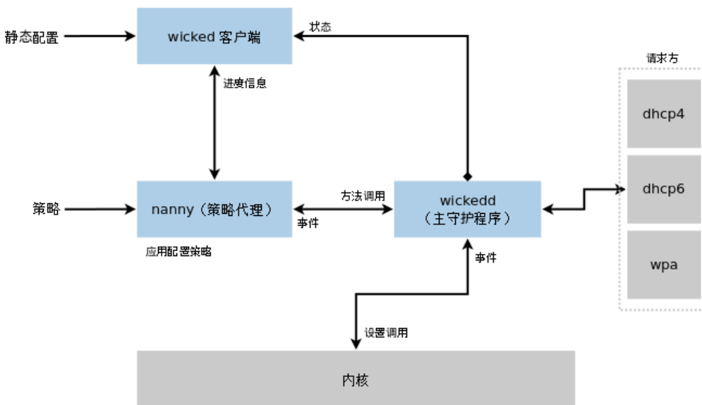
图 16.4 : wicked 体系结构
