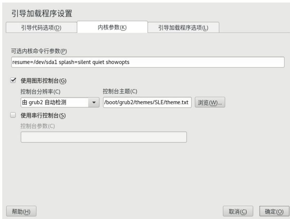
图 12.4：内核参数
