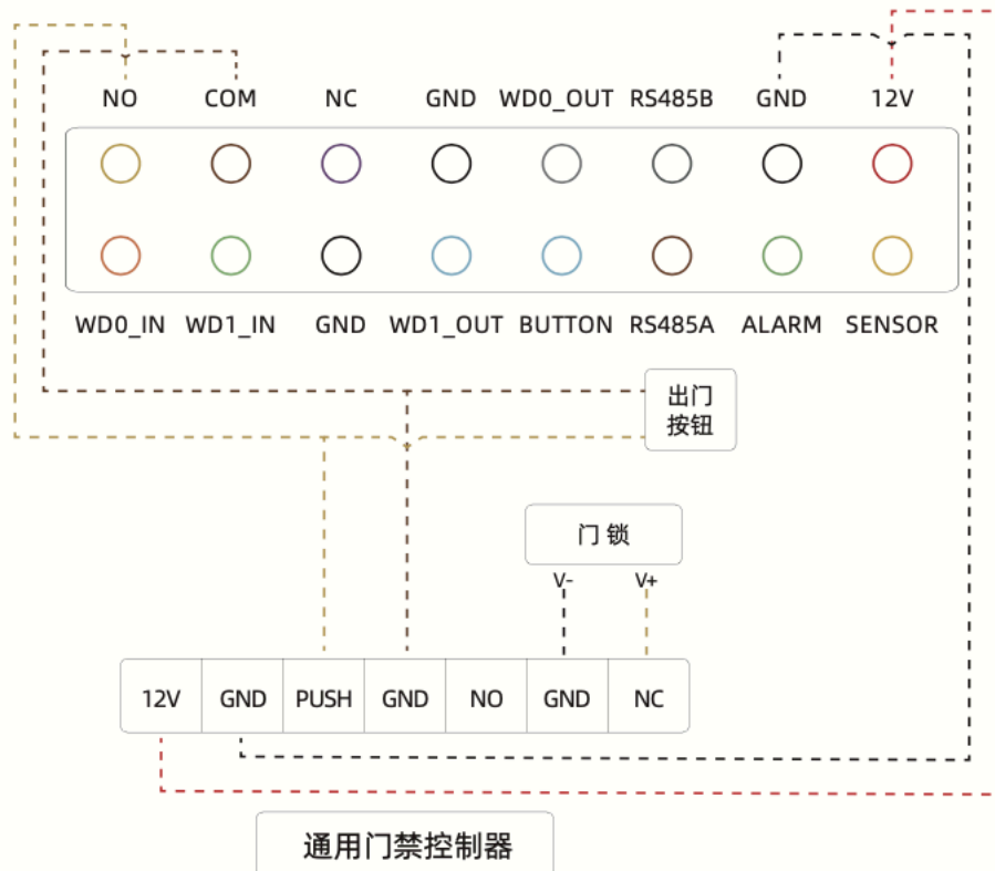
图 3-1-5 Y3s 设备接线示意图
