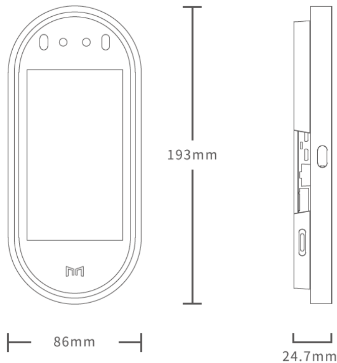
图 1-4-1 产品尺寸
