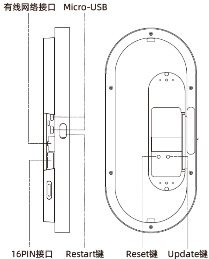
图 2-1-2 左侧及背面布局图
