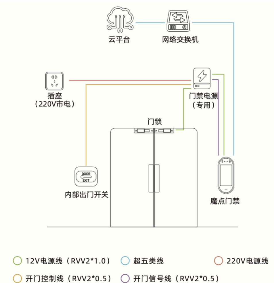
图 3-1-1 系统拓扑图
