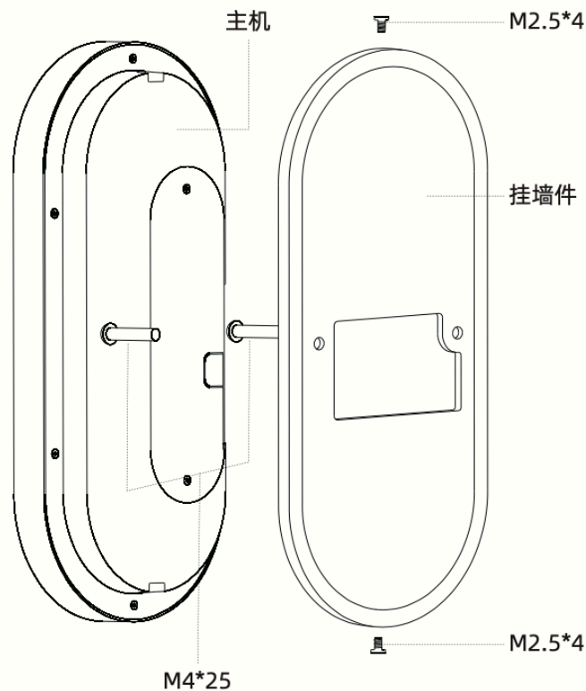
图 3-1-2 安装示意图
