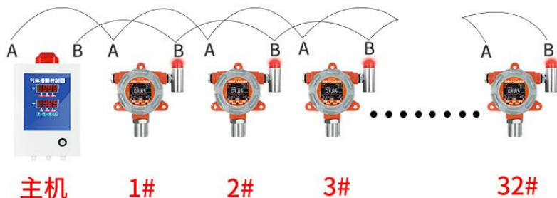
手拉手布线图
