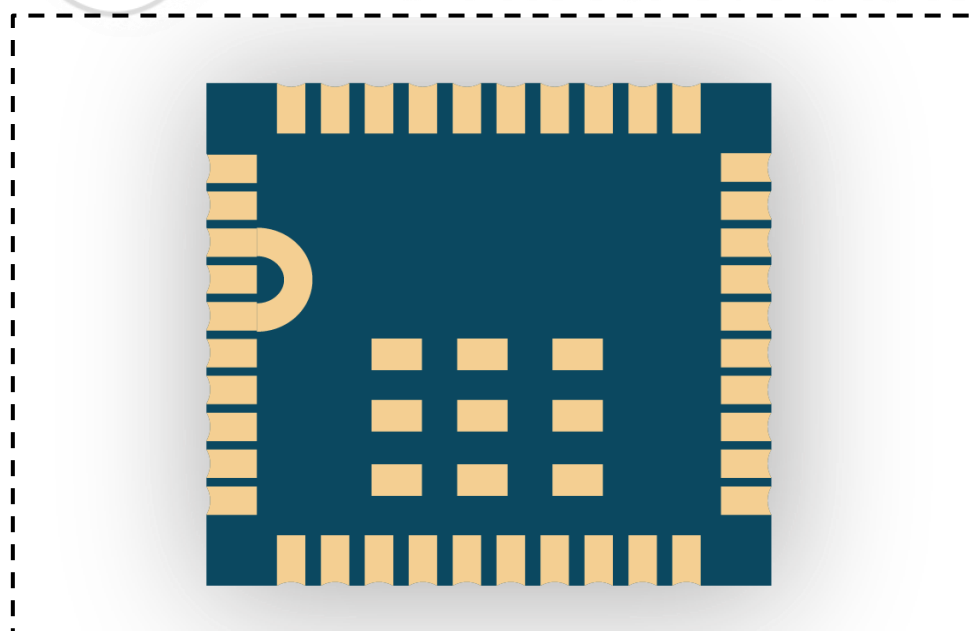
图 24：模组底视图
